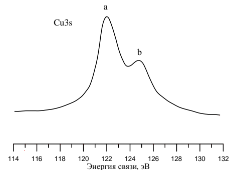
Рис.17 Рентгеноэлектронный Cu3s спектр жидкой меди.
