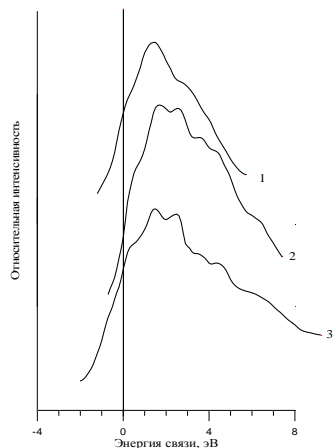
Рис.14. Рентгеноэлектронные спектры валентных полос: 1 - Mn, 2 - Fe, 3 - Fe_{50}Mn_{50} ( T=300K ).
