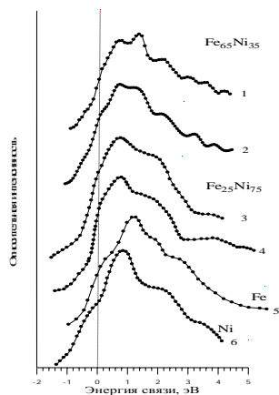
Рис.9. Рентгеноэлектронные спектры валентных полос эталонов: 5 – Fe, 6 – Ni и сплавов: 1 – Fe_{65}Ni_{35} при T_{комн.} , 2 – Fe_{65}Ni_{35} при T=500K ; 3 – Fe_{25}Ni_{75} при T_{комн.} , 4 – Fe_{25}Ni_{75} при T=870K .
