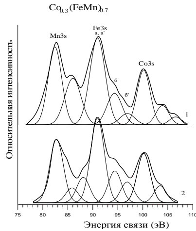
Рис.15. Рентгеноэлектронные 3s- спектры Mn, Fe и Co сплава Co_{0.3}(FeMn)_{0.7} в: 1- антифер. сост.(T=300K), 2 – парамаг. сост.(T=300K)
