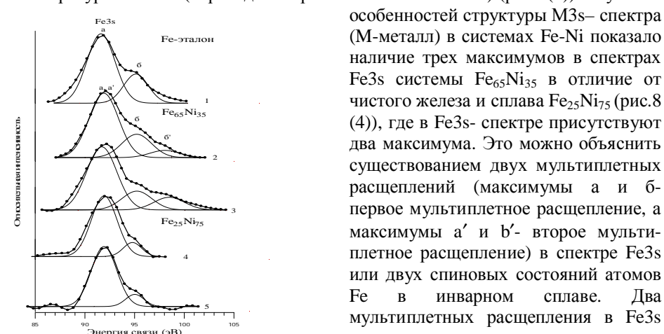
Рис.8. Рентгеноэлектронные Fe3s-спектры: 1- чистого Fe; 2 – сплава Fe 65 Ni 35 при T комн. , 3- Fe 65 Ni 35 при T=500K; 4 – сплава Fe 25 Ni 75 при T комн. , 5- Fe 25 Ni 75 при T=870K.
