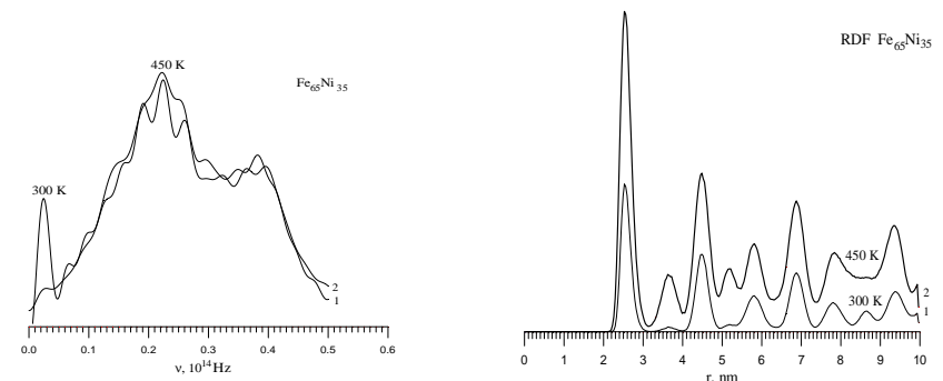
Рис.11. Плотность колебательных состояний атомов в Fe_{65}Ni_{35} при а) 300К, б) 500К.
