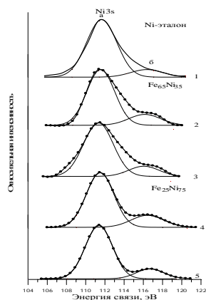
Рис.10. Рентгеноэлектронные Ni3s -спектры: 1 – чистого Ni; 2 – Fe_{65}Ni_{35} сплава при T_{комн.} , 3 – Fe_{65}Ni_{35} при T=500K ; 4 – Fe_{25}Ni_{75} сплава при T_{комн.} , 5 – Fe_{25}Ni_{75} при T=870K .
