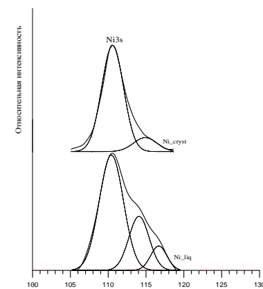
Рис.18. Ni3s -PЭ спектры в: а) кристаллическом состоянии (300 К); б) жидком состоянии (1800 К).
